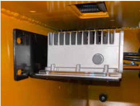
On-Board-Ladegerät
